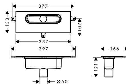
uBox universal za vertikalnu instalaciju
