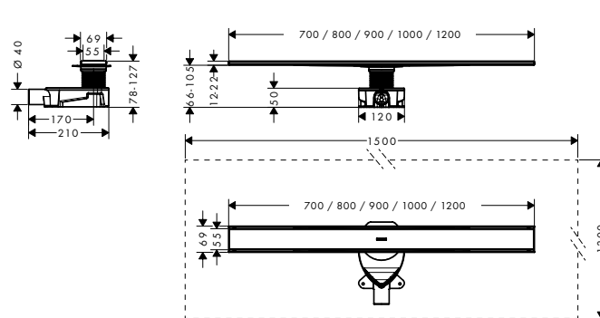
RainDrain Allround ravna instalacija
