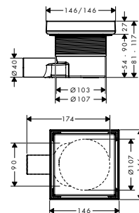
RainDrain Point sa popločivom rešetkom 150 x 150
