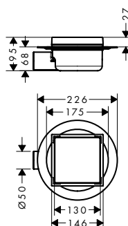
RainDrain Spot sa popločivom rešetkom
