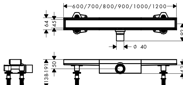
RainDrain Compact ravna instalacija
