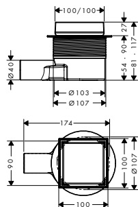
RainDrain Point sa popločivom rešetkom 100 x 100
